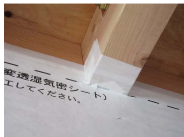
胴差に30mm重ね気密テープ張り
